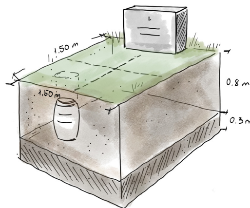
Illustrasjonen viser utforming av urnegrav.
