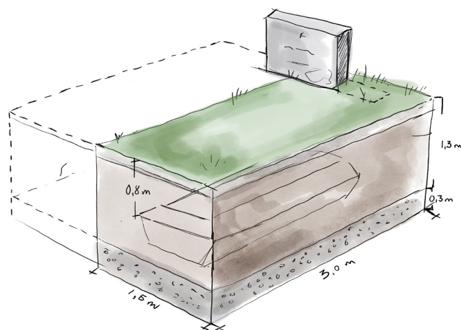
Illustrasjonen viser utforming av kistegrav.
